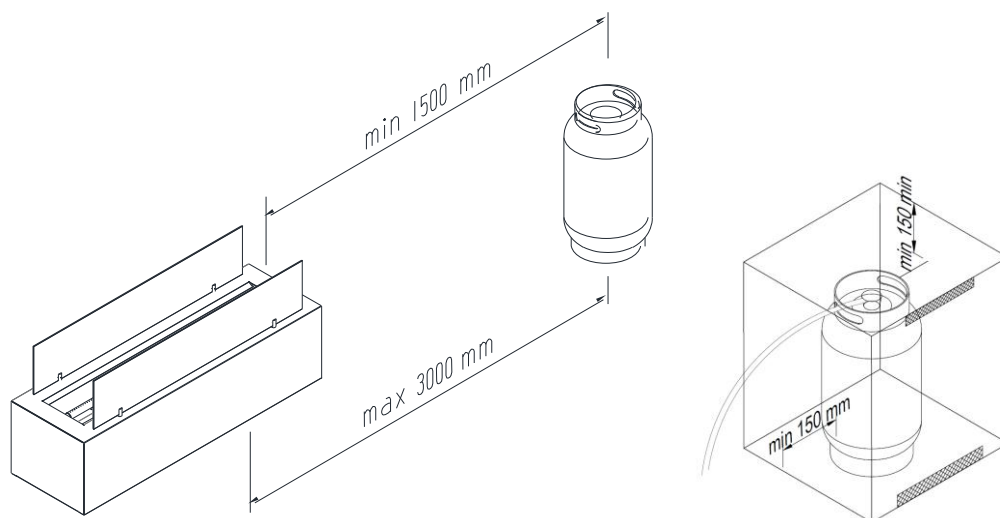
Abbildung 2 – Abstand zwischen der Feuerstelle und Gasflasche sowie Gasflaschenverkleidung
