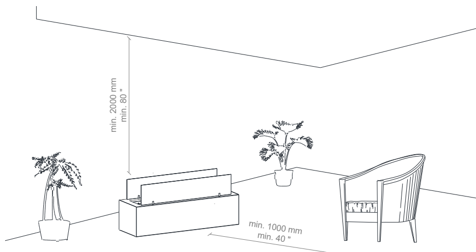
Abbildung 1: Mindestabstand zu brennbaren Materialien
